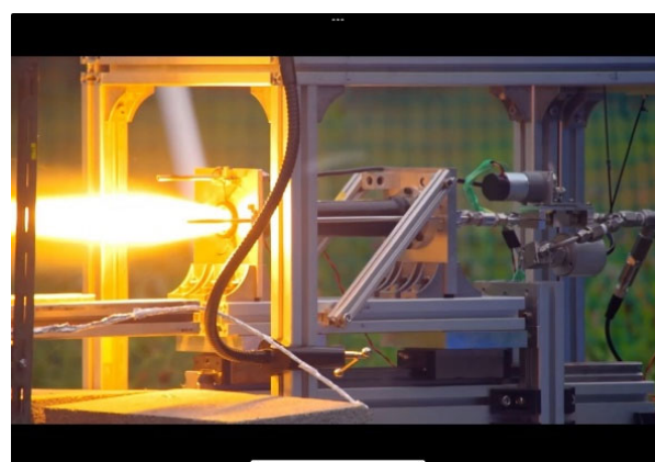
(自作燃焼システムの燃焼実験)
